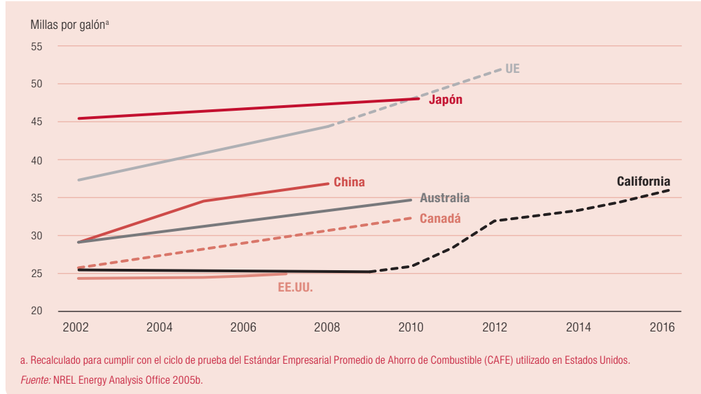
Figura 3.5 Las normas de eficiencia sobre combustibles difieren mucho en los países desarrollados
