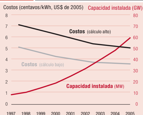
Figura 3.4 Energía eólica en EE.UU.: su capacidad aumenta y los costos disminuyen
