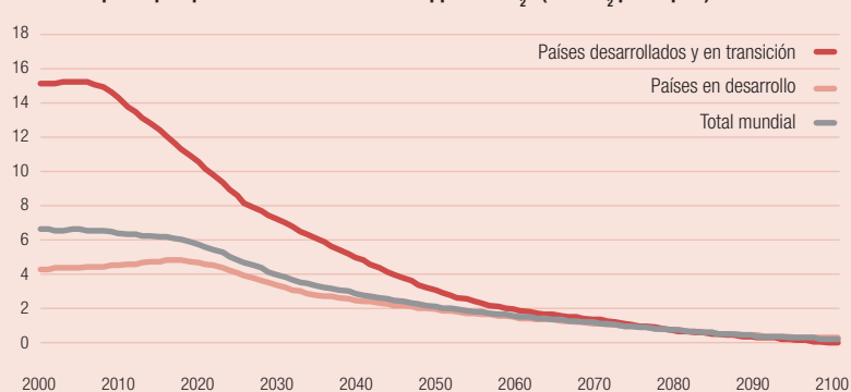
Figura 1.12 Contracción y convergencia hacia un futuro sostenible
