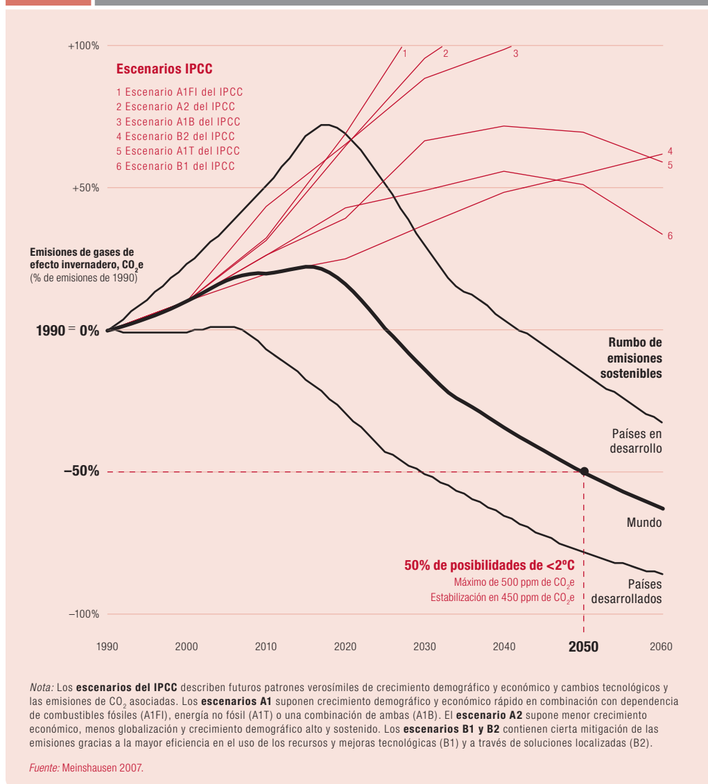
Figura 1.11 Reducir las emisiones a la mitad antes de 2050 podría evitar el cambio climático peligroso
