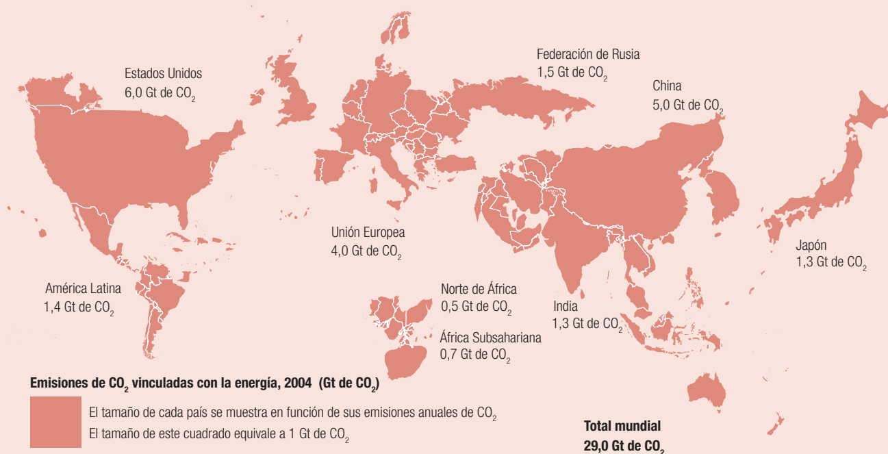
Representación de la variación mundial de emisiones de CO 2
